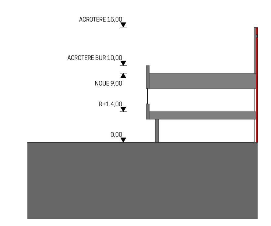
COUPE EE
