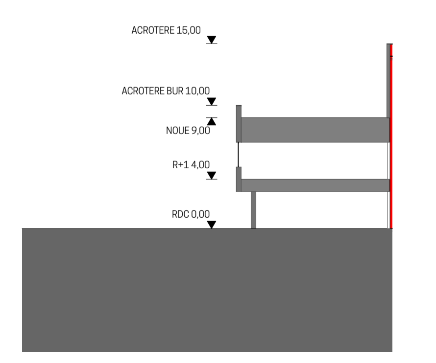
COUPE DD
