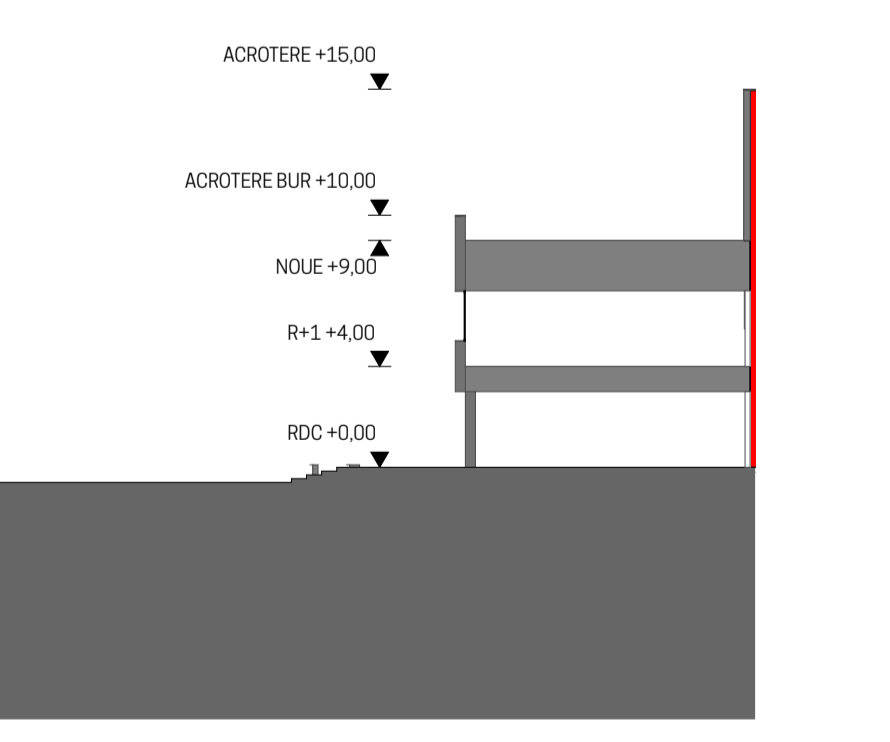
COUPE CC
